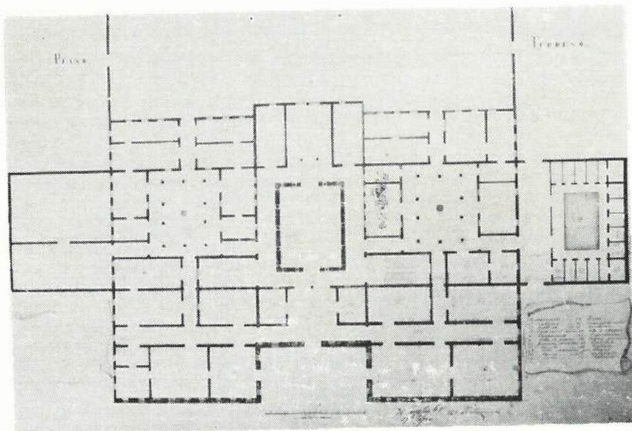
Slika br. 8. Projekt Perikla Koludrovića nove Bolnice u Splitu, neizvedeno, iz 1868. god. (prizemlje)
