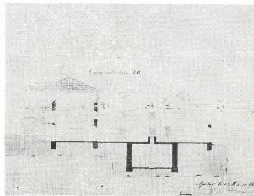
Slika br. 5. Projekt Ivana Lucchinija za proširenje Bolnice u Splitu, neizvedeno, iz 1841. god. (poprečni presjek)
