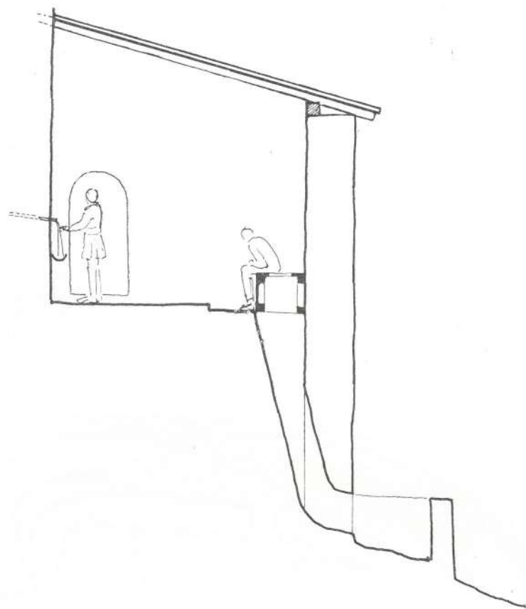
Rekonstrukcija latrine
